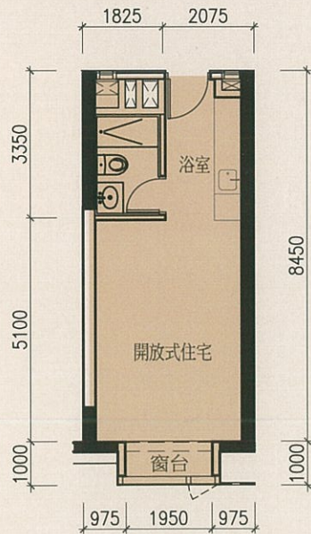
H、J、L、N 及 P 單位平面圖 469 平方呎
