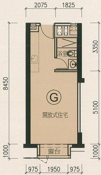
G 單位平面圖 466 平方呎
